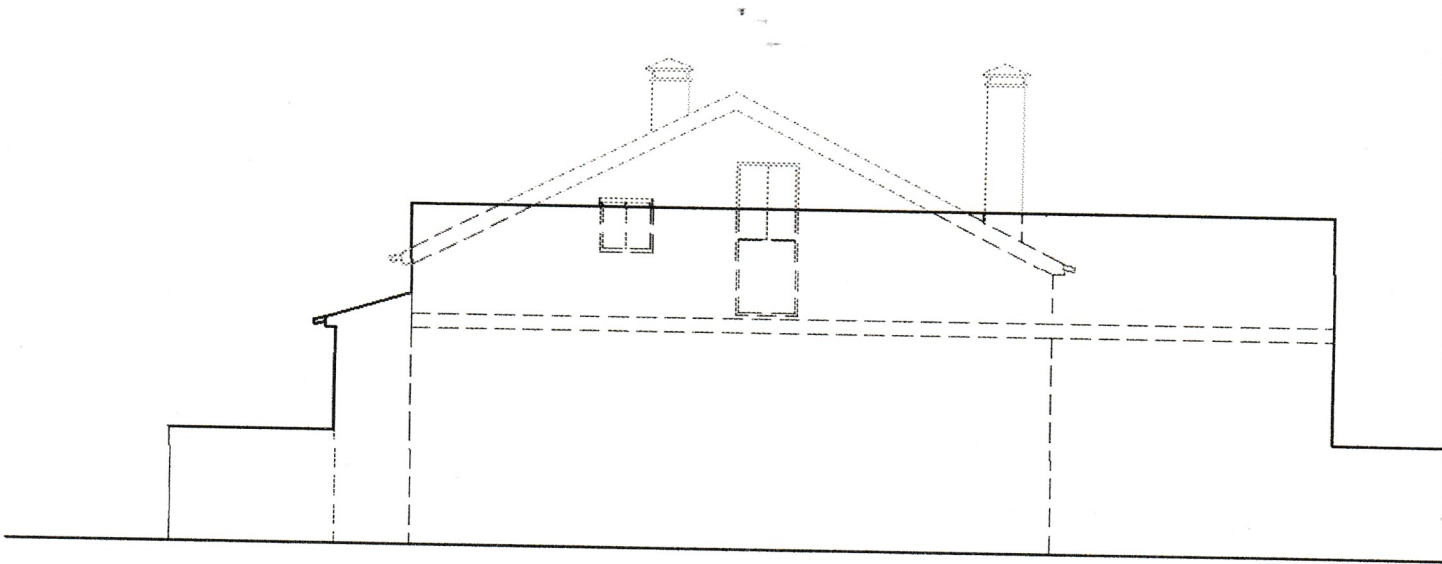
ALÇADO PRINCIPAL
